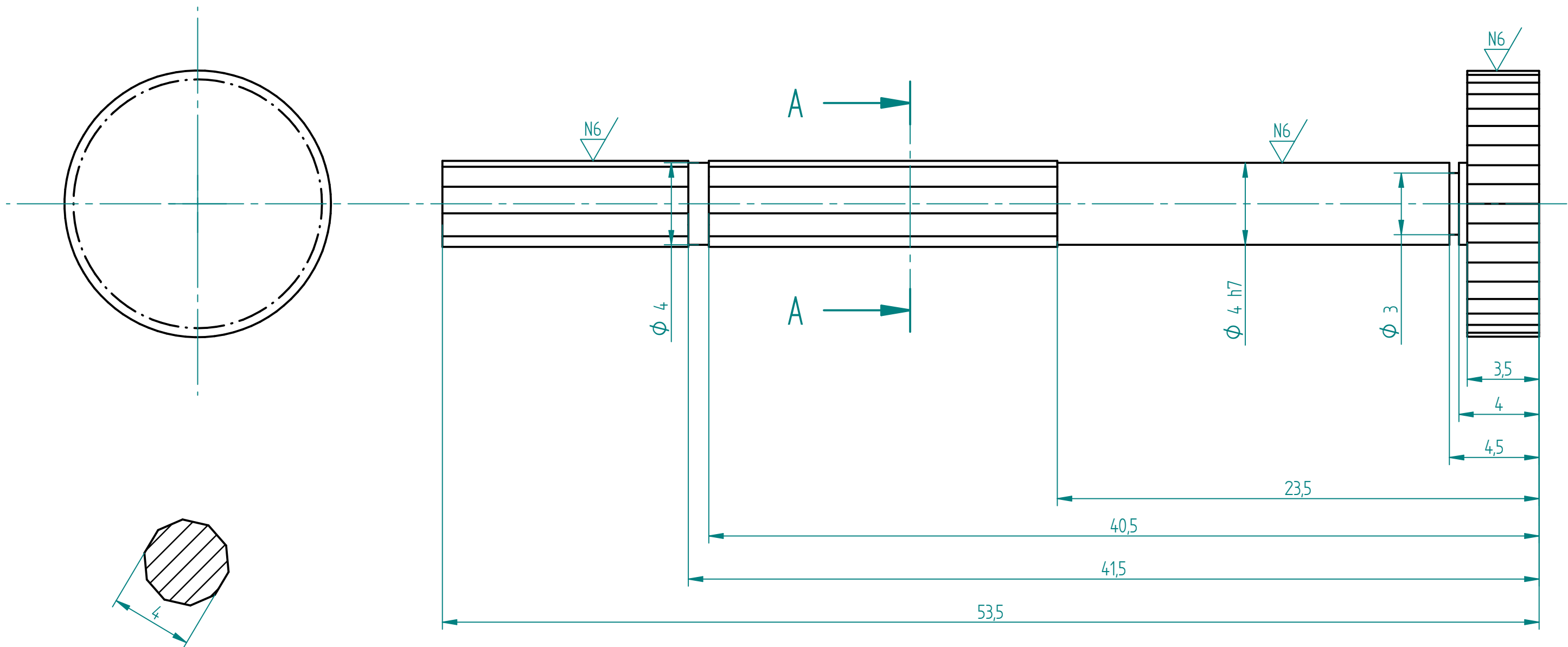
A-A EBAKETA
